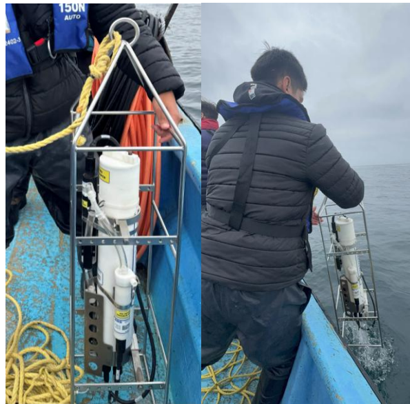
Figura 3 Equipo CTD Seabird® 19 empleado para el estudio de la salinidad y temperatura en la columna de agua.
